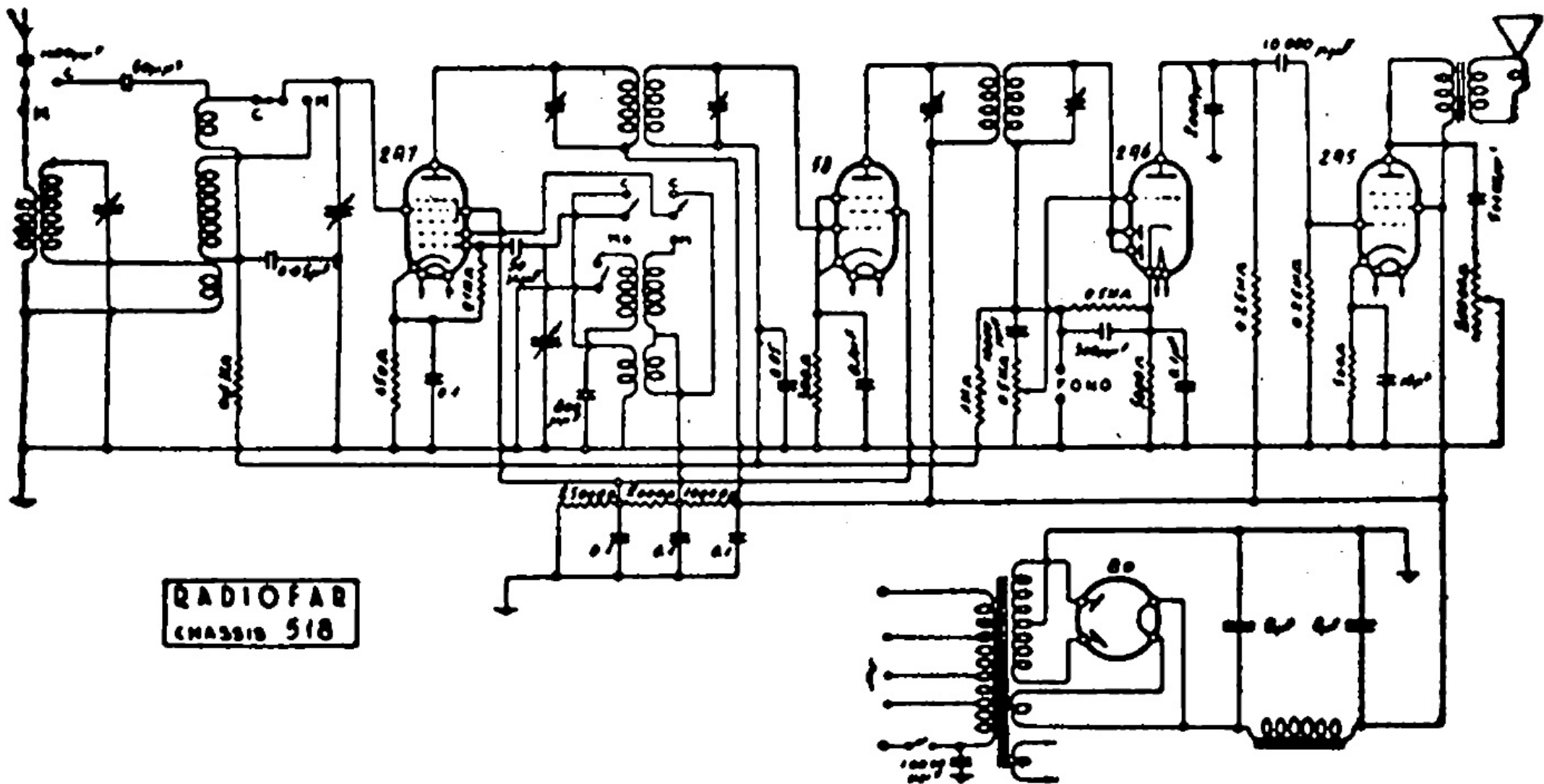
S. A. RADIOFAR — Modello «Chassis 518» — Produzione 1936. — Media frequenza: 175 mc.
